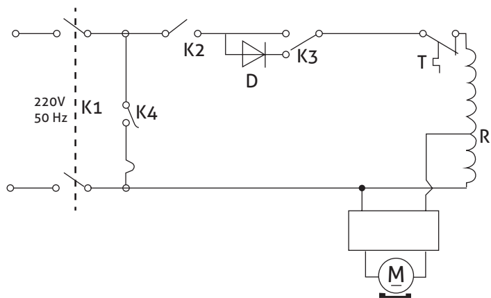
Diagrama de electricidad
